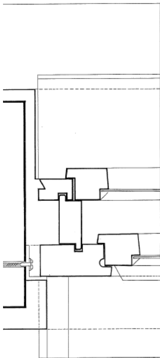
PLAN (KASA + KANAT)
